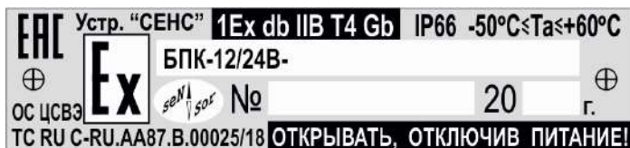
Табличка поз.11
