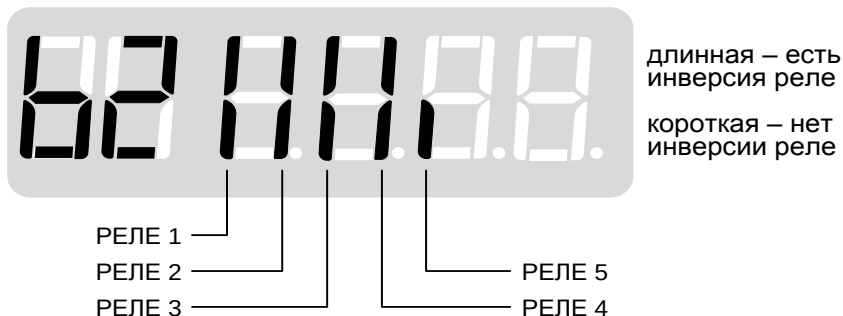
Рисунок 8 – Пример табло показывающего прибора при внесении записи параметра b2
